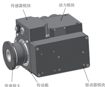
图2 腕部平台外形图
