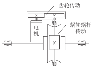
图3 腕部平台传动简图
