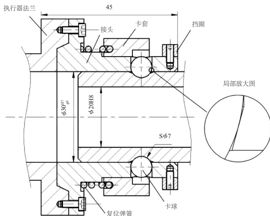
图6 快速接头结构图
