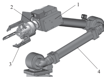
1—臂上腕部平台;2—快速接头; 3—末端执行器模块(图示为夹持模块);4—机械臂 图1 机械臂与可更换末端执行器结构三维模型
