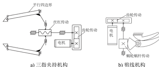
图5 末端执行器机构简图
