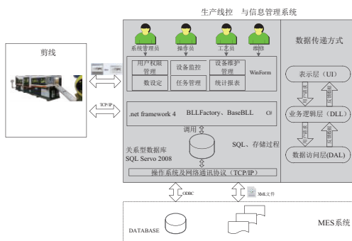
横剪线控制及信息管理系统的主要功能结构由用户权限管理模块、设备控制模块、任务管理模块、生产统计模块等组成,其功能模块如图 5 所示。其中用户权限管理模块主要对系统使用人员信息和权限进行管理;设备操作模块主要包括横剪线设备监控、参数设置、片型管理、任务管理等功能;设备维护模块主要进行集中监视、管理设备的定期维护事项(如日检修、周检修、月检修、半年检修以及刀具使用寿命情况等)。生产统计模块主要是对变压器铁心生产任务的完成量、每天生产硅钢片量、设备开机率等信息进行统计,并可按指定报表格式输出。故障诊断模块主要是侦测 PLC、伺服电机、变频器以及系统逻辑故障信息,并进行记录保存,便于后续追溯查询。
