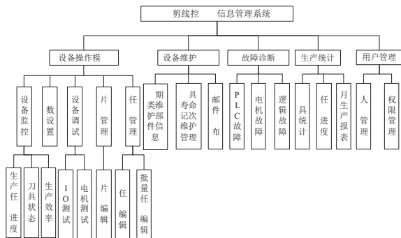
横剪线控制及信息管理系统的主要功能结构由用户权限管理模块、设备控制模块、任务管理模块、生产统计模块等组成,其功能模块如图 5 所示。其中用户权限管理模块主要对系统使用人员信息和权限进行管理;设备操作模块主要包括横剪线设备监控、参数设置、片型管理、任务管理等功能;设备维护模块主要进行集中监视、管理设备的定期维护事项(如日检修、周检修、月检修、半年检修以及刀具使用寿命情况等)。生产统计模块主要是对变压器铁心生产任务的完成量、每天生产硅钢片量、设备开机率等信息进行统计,并可按指定报表格式输出。故障诊断模块主要是侦测 PLC、伺服电机、变频器以及系统逻辑故障信息,并进行记录保存,便于后续追溯查询。
