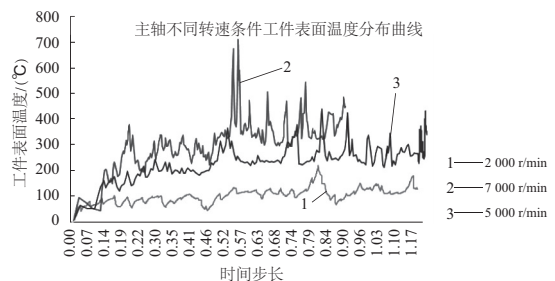
图 6 不同主轴转速下被加工表面温度分布随时间变化曲线图
